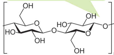
Cellulose
